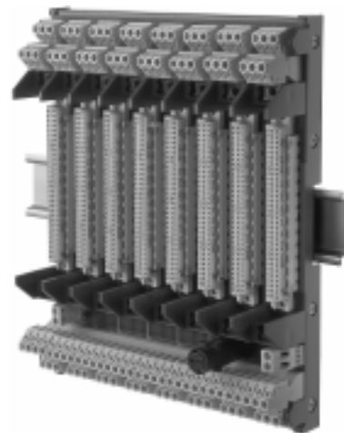
BP 902-28 mit 8 Steckplätzen
